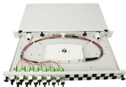
Beispielbestückung E2000
