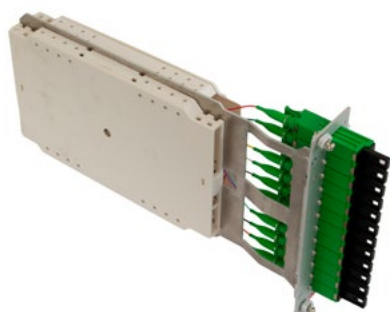
E2000-Bestückung
